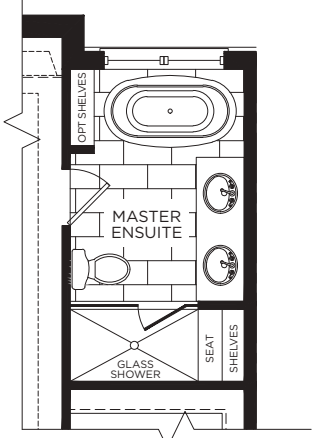
Opt Master Ensuite Layout
